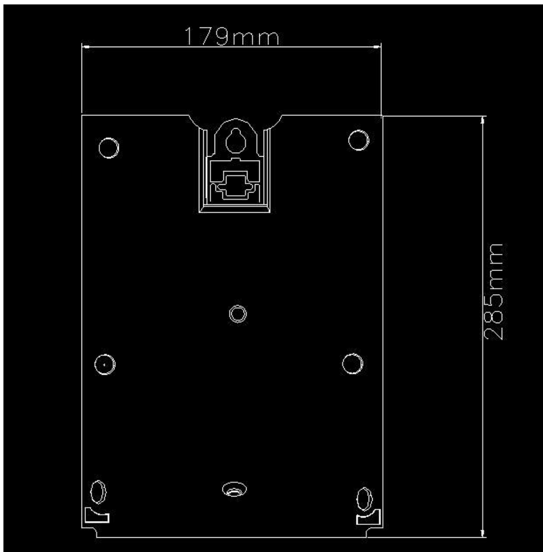
图 四 安装孔位
