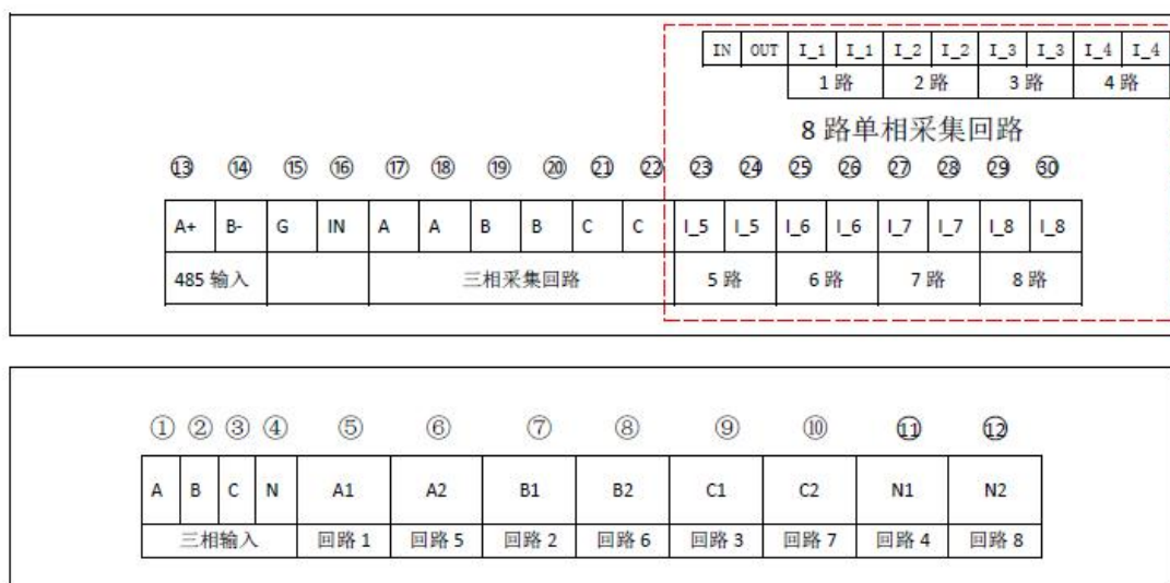
图 五 接线图
